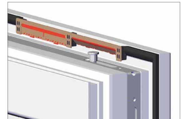
Sistema di aerazione nella zona di battuta della finestra arimeo – Il sistema di aerazione invisibile
