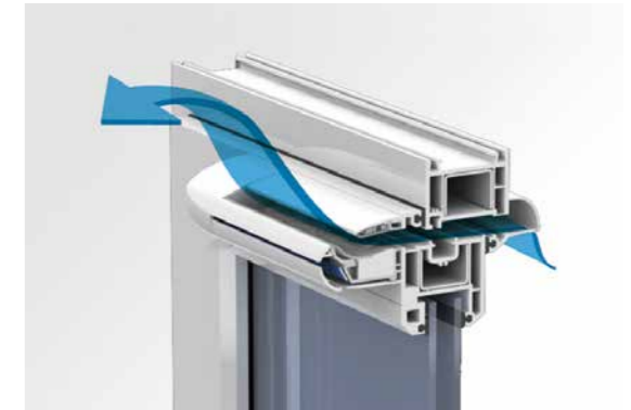
SECCO-Plus – Il semplice sistema di diffusione dell'aria esterna
