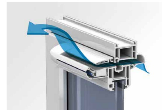
SECCO-Plus – le système simple d'évacuation d'air
