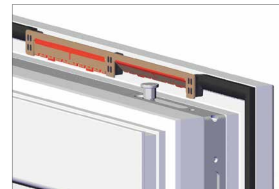
Aérateur de feuillures de fenêtre arimeo – le système de ventilation simple et invisible
